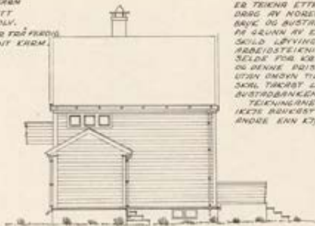
RUSTFASADE.
